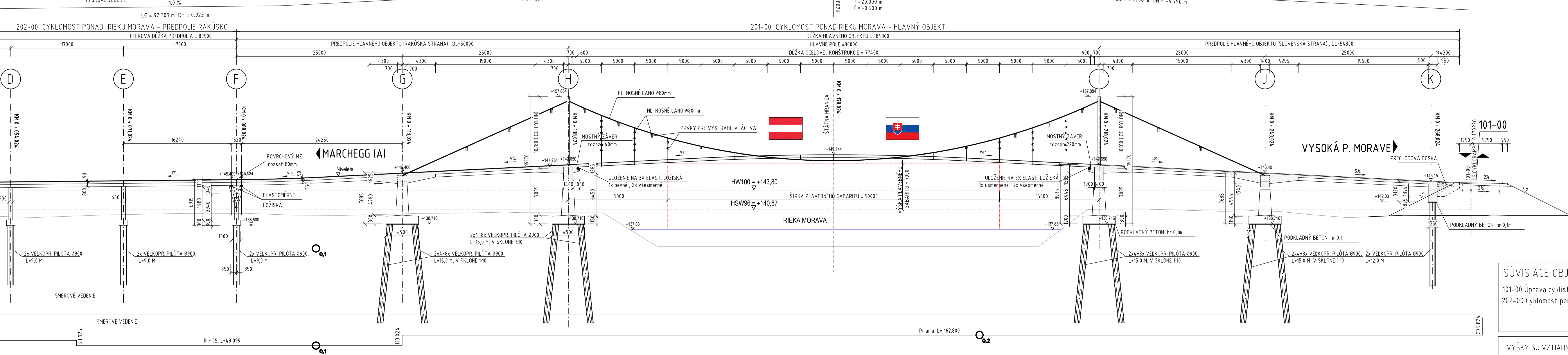
POZDĽŽNÝ REZ M 1:250
